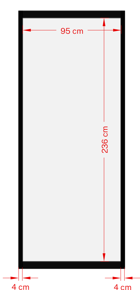
Prospetto
